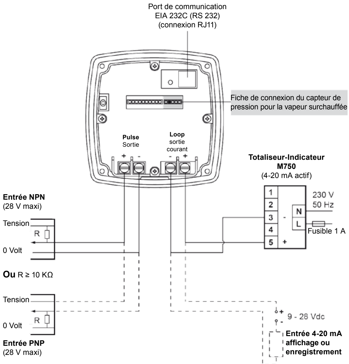
Fig. 20 - Schéma de câblage du TVA avec communications EIA 232 (RS232) et 4-20 mA.
