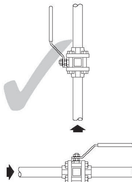
Fig. 3 Installation correcte pour les applications gaz
