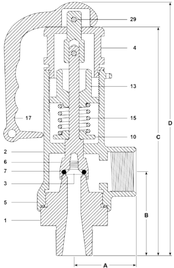
Fig. 2 - SV405, SV406 et SV405X
