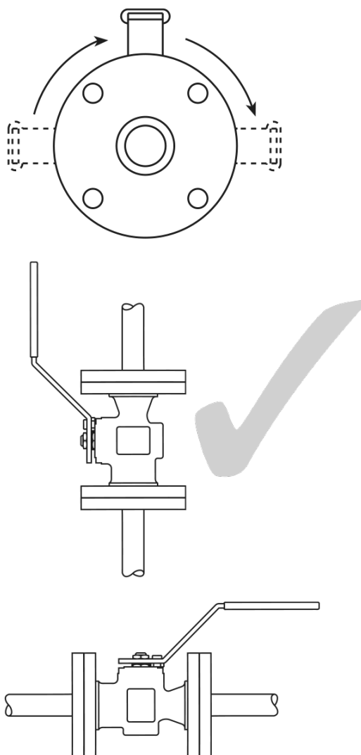
Fig. 3 - Installation correcte pour les applications de gaz
