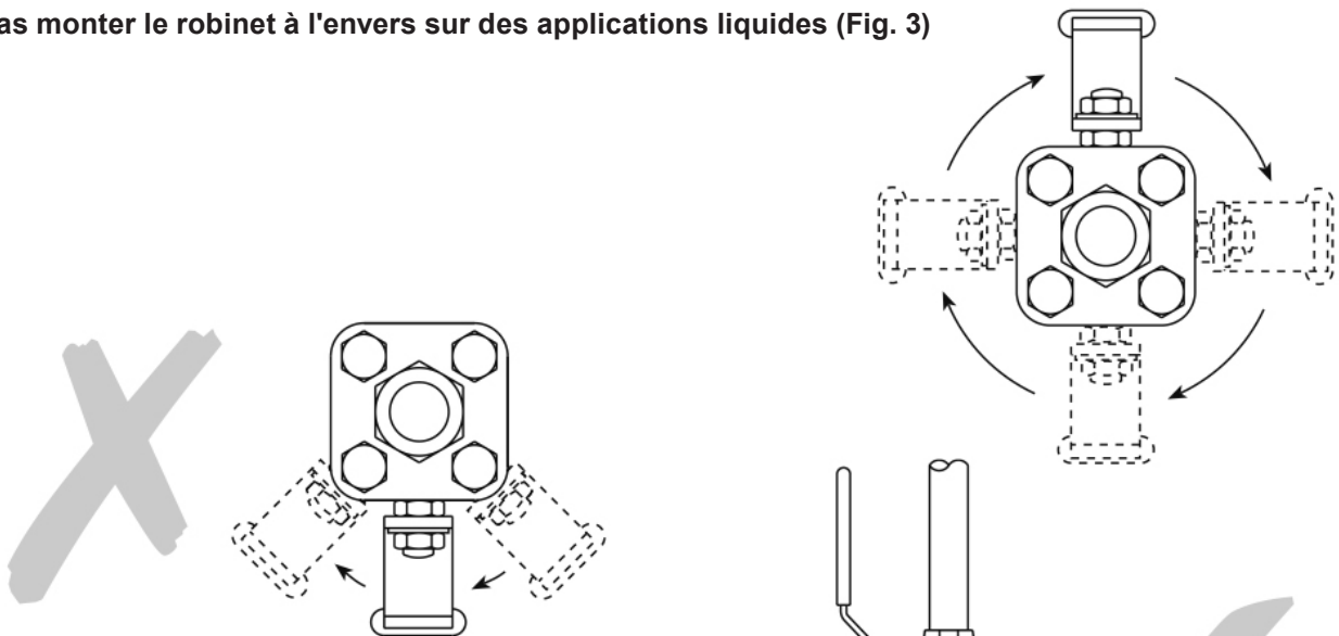
Fig. 3 - Installation incorrecte pour les applications liquides
