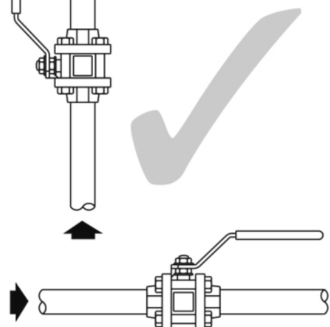
Fig. 4 - Installation correcte pour les applications gaz
