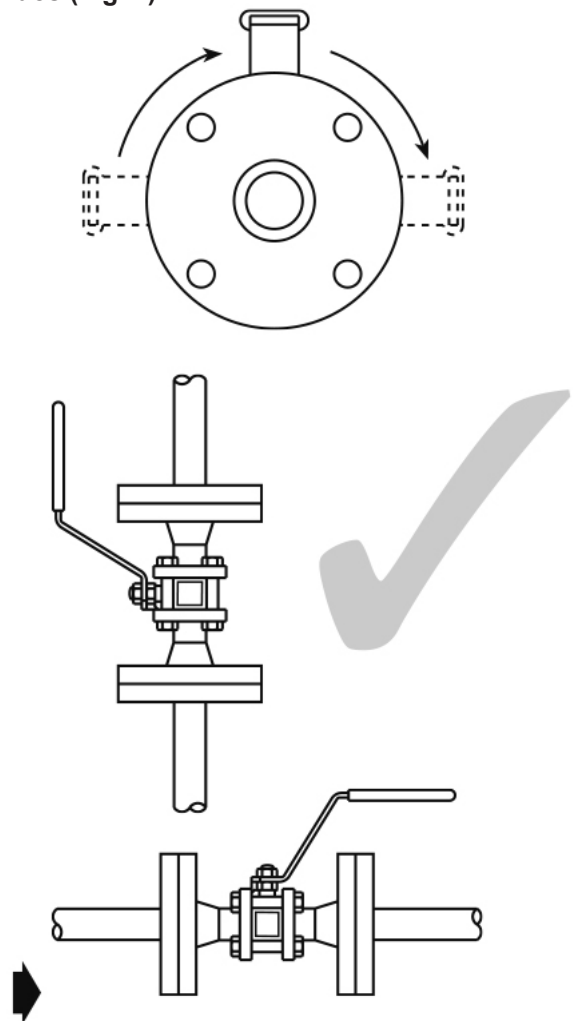
Fig. 3 Installation correcte pour les applications gaz
