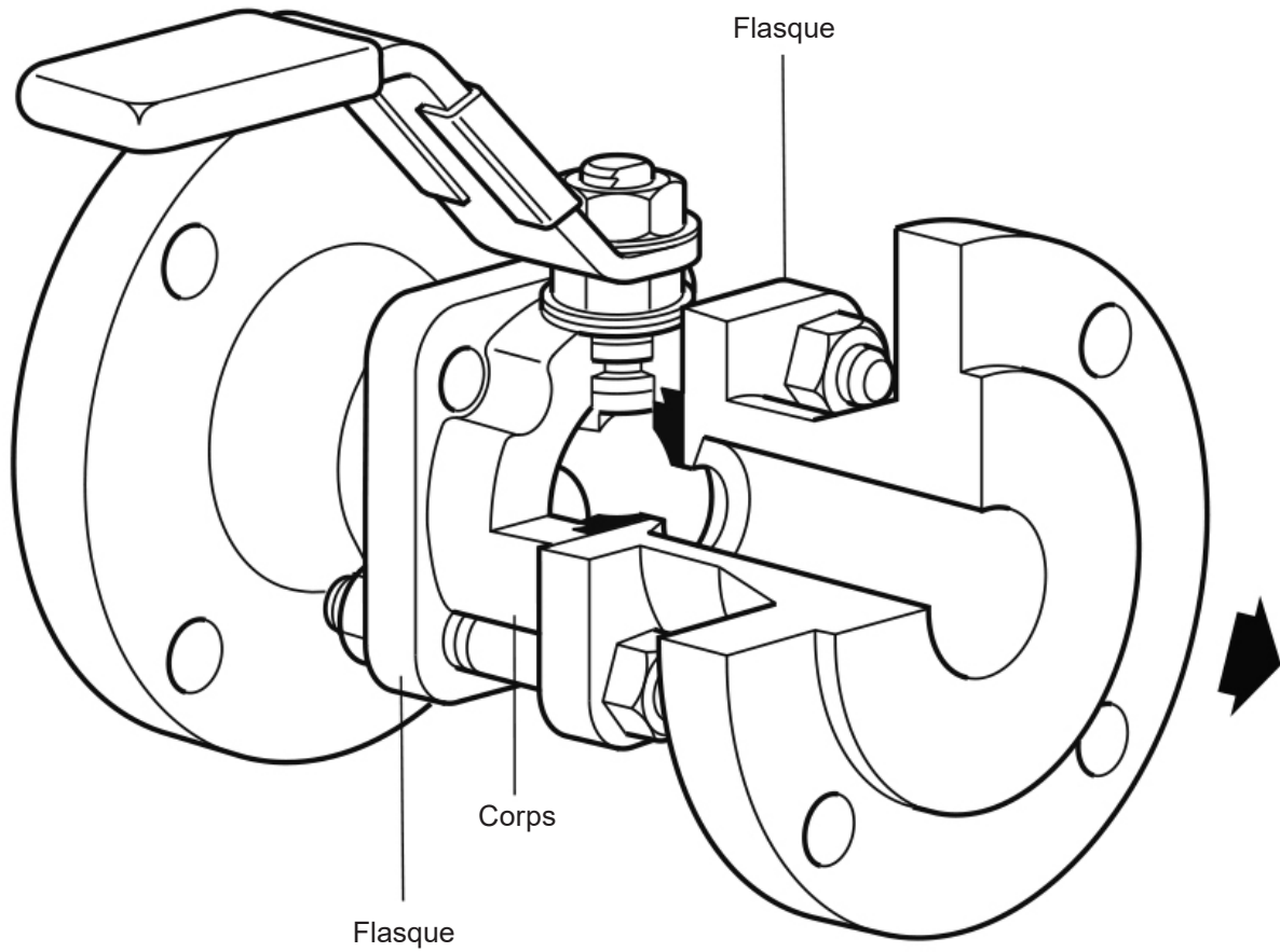
Fig. 1 - M10ECF - Version à brides
