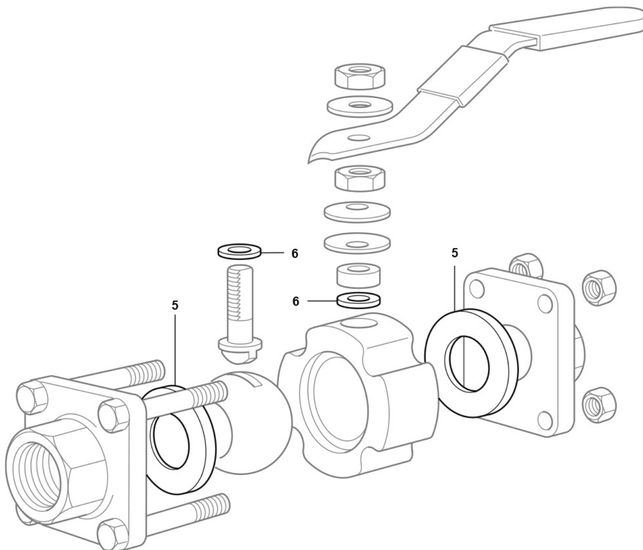
Fig. 5 - M10ECF - Version taraudée
