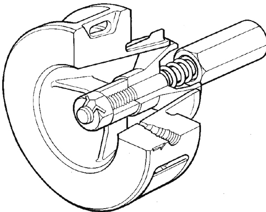
Fig. 2 - ILVA DN200
