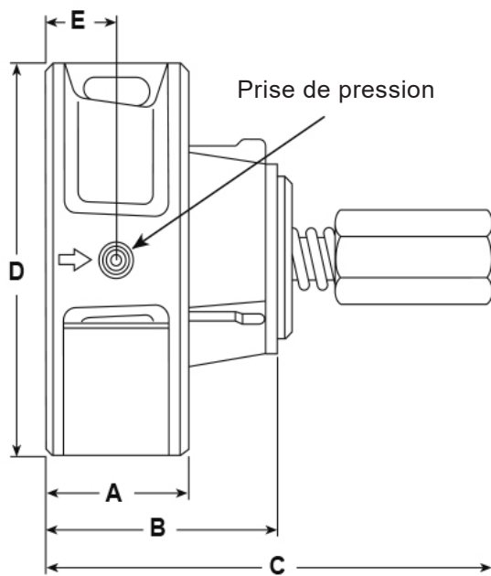
Fig. 3 - ILVA DN50 - DN200
