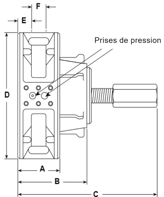
Fig. 4 - ILVA DN250 - DN300
