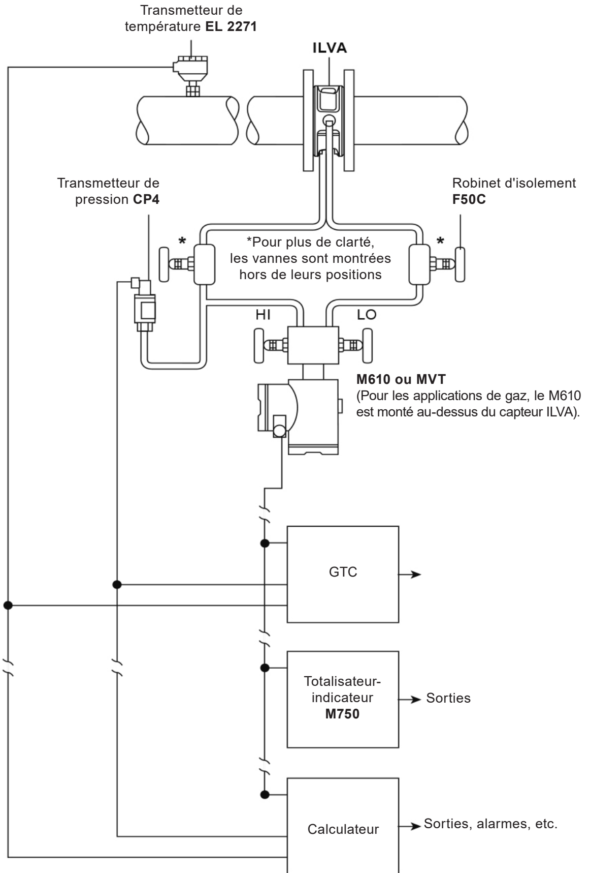
Fig. 1 (Schématique uniquement) Voir Fig. 15 pour les détails
