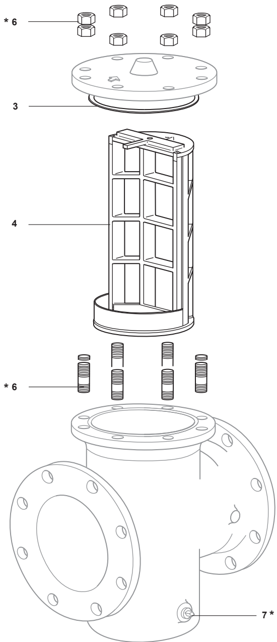
Filtre à panier Fig 7
