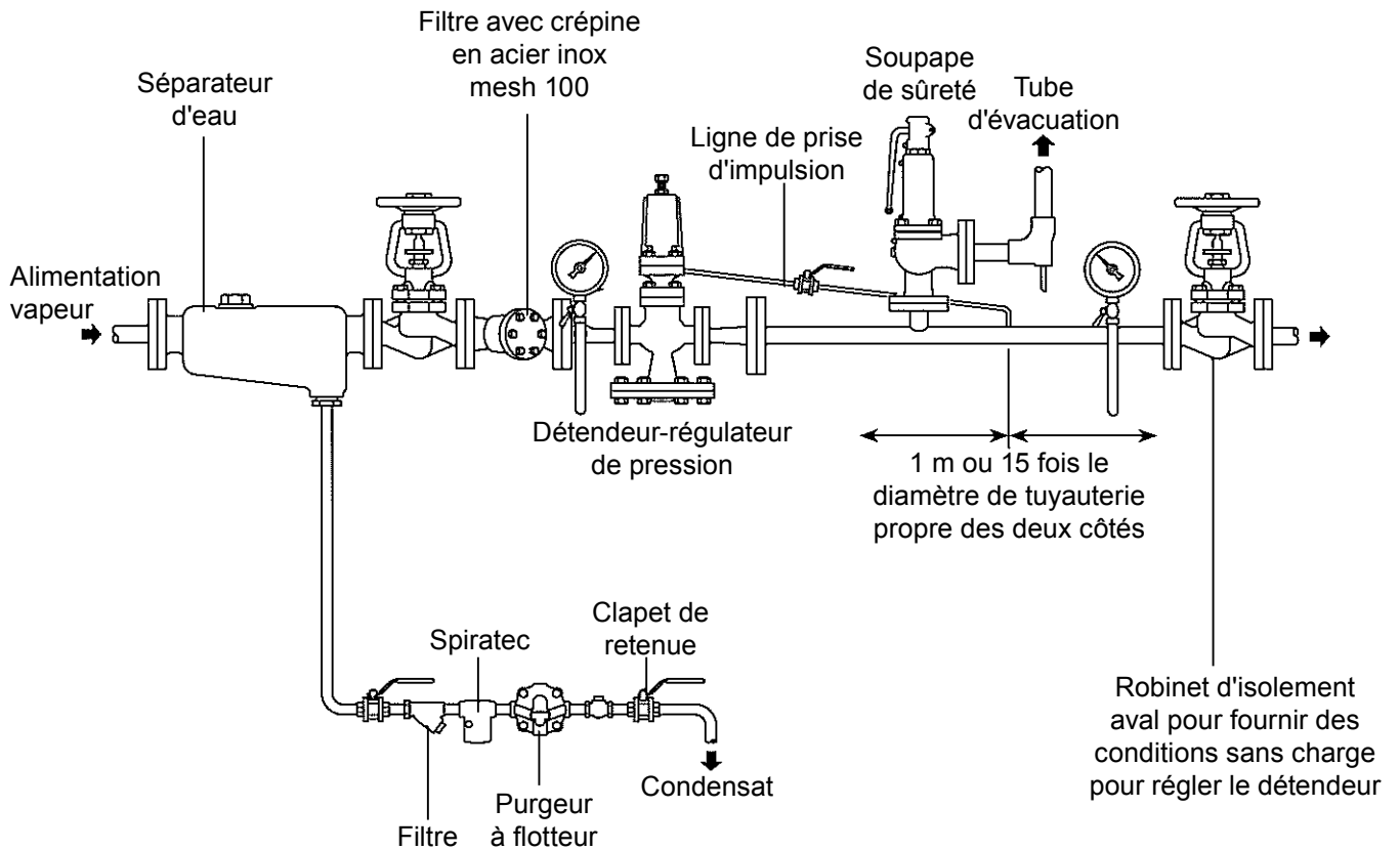
Fig. 2 Installation recommandée
