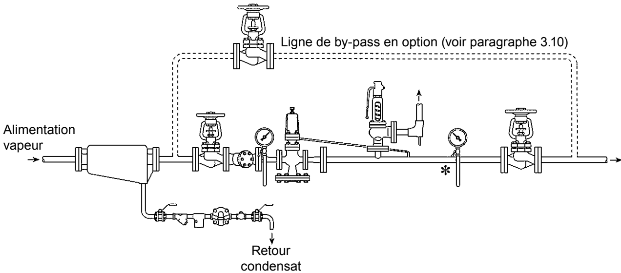
Fig. 4 DP143, DP143G et DP143H - Procédure de réglage
