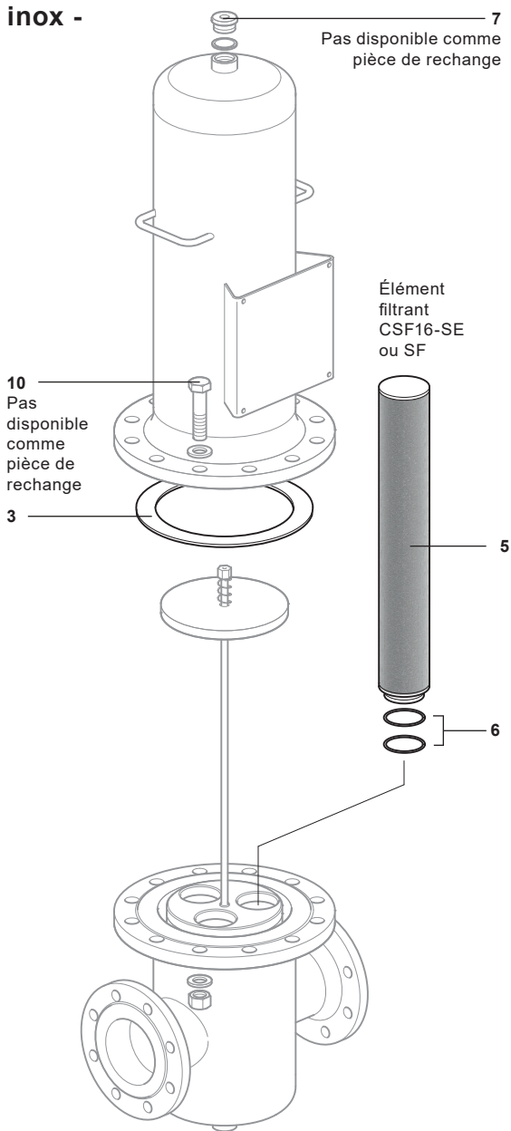
Fig. 12 DN100 et DN150L (l'image représente un DN100L)
