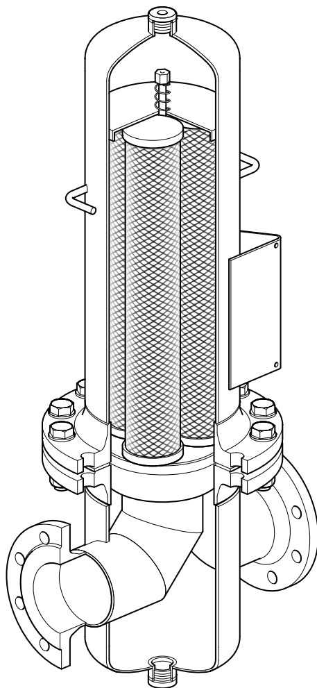
DN100 et DN150
