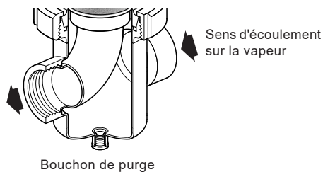
Fig. 3 Filtre à vapeur - DN8 à DN80
