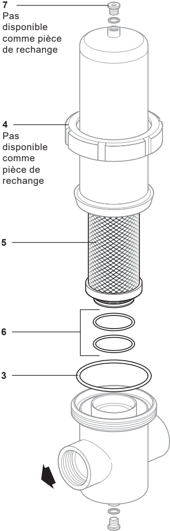
Fig. 13 DN8 au DN80
