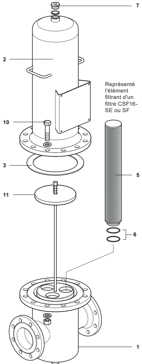
Fig. 8 Filtre à vapeur - DN100 et DN150 (Représenté DN100L)
