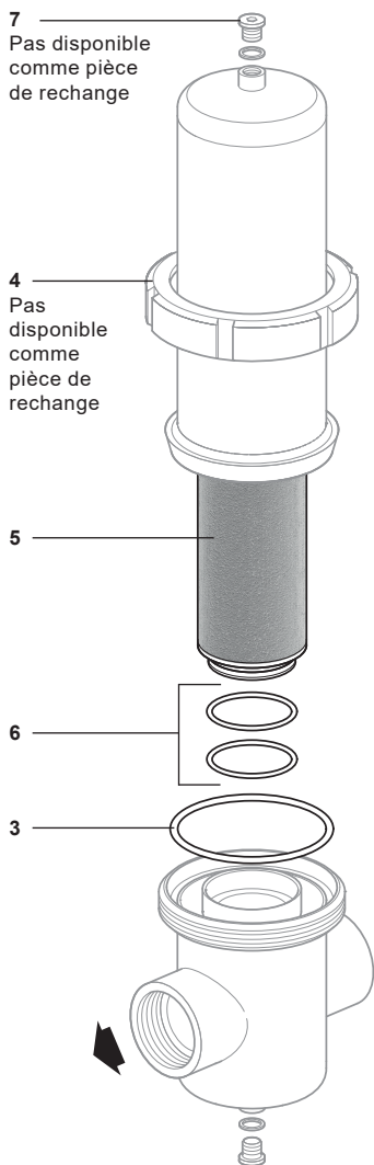
Fig. 11 DN8 au DN80
