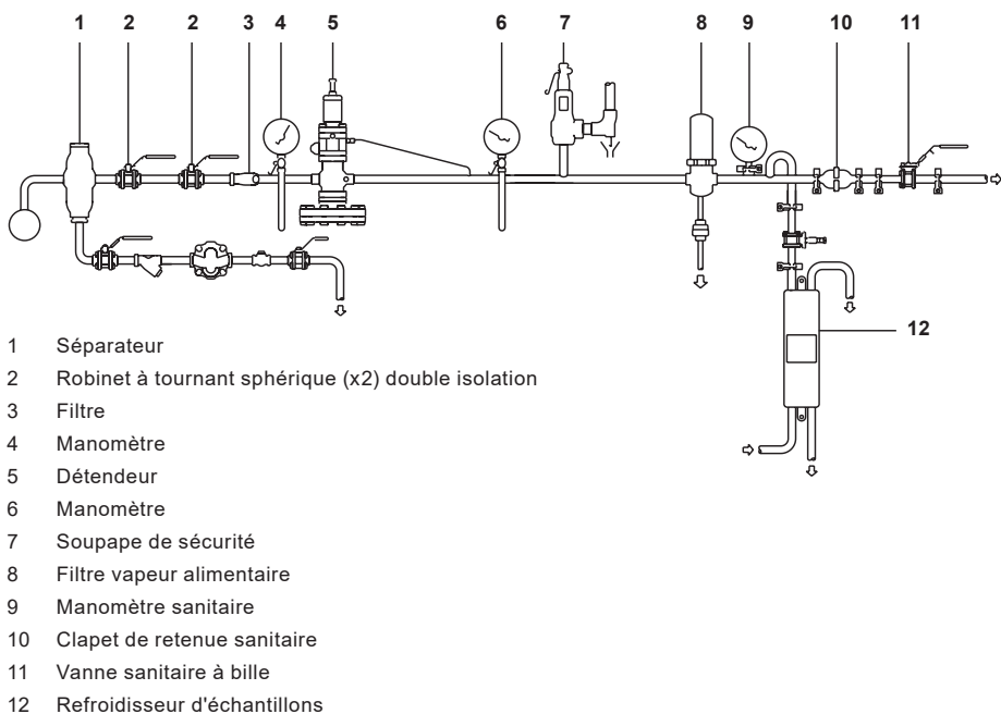
Fig. 2 - Station de vapeur filtrée typique
