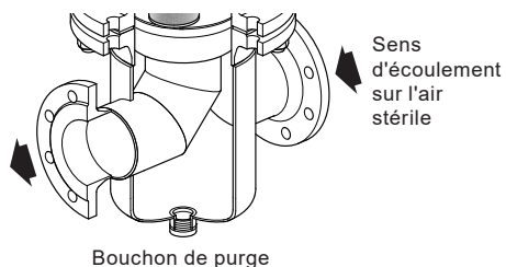
Fig. 4 Filtre à vapeur - DN100 et DN150
