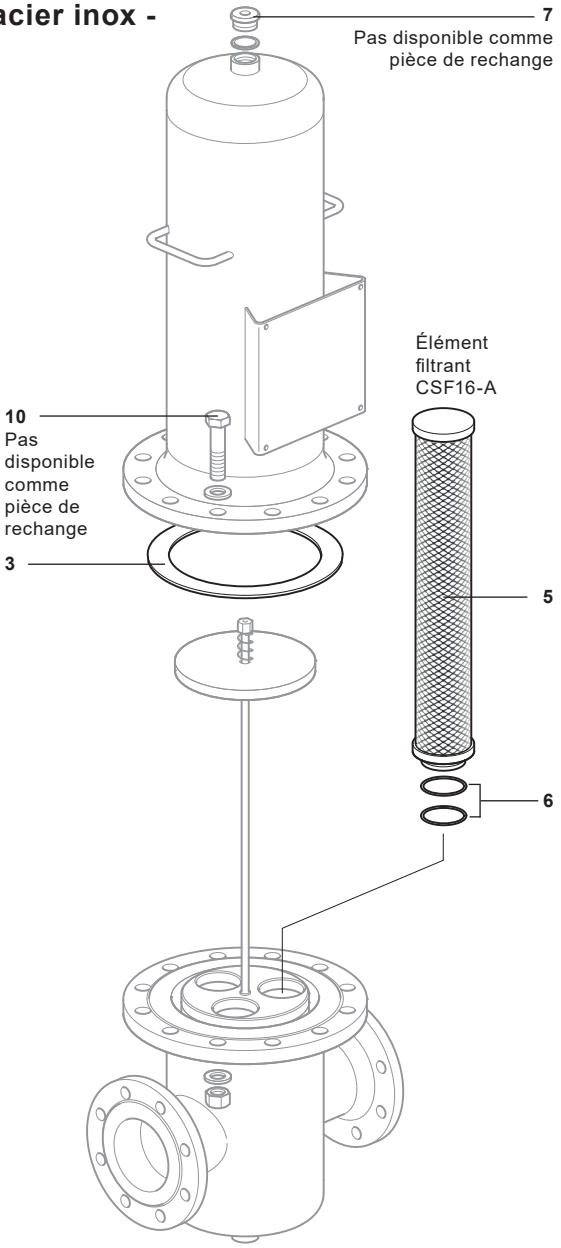
Fig. 14 DN100 et DN150L (l'image représente un DN100L)
