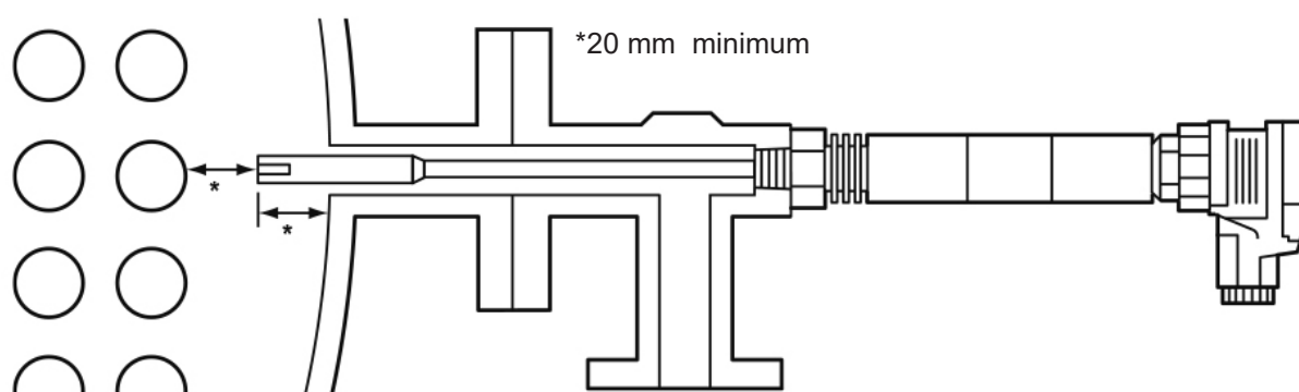
Fig. 2 - Installation type montrant une sonde montée dans un coude de sonde
