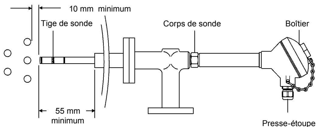
Fig. 2 - Schéma d'installation
