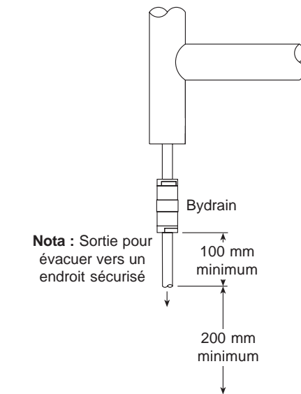
Fig. 4 - Montage vertical
