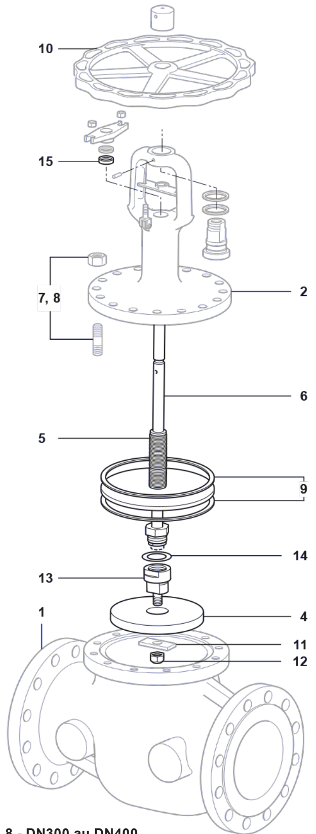
Fig. 8 - DN300 au DN400
