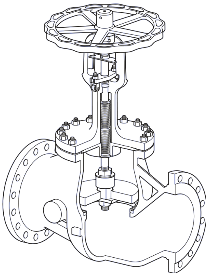
Fig. 2 - Robinets à soupape à soufflet BSA3-BD DN300 et DN400
