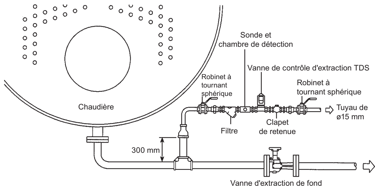
Fig. 4 Installation en parallèle sur l'extraction de fond de chaudière
