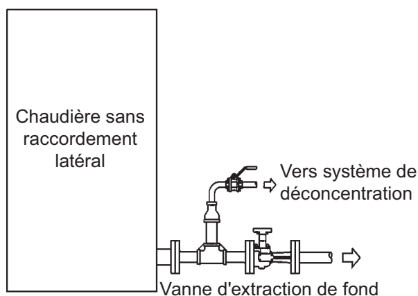
Fig. 3 Raccordement du système de déconcentration avec raccordement en 'T'
