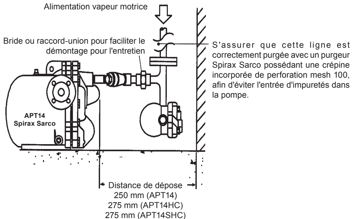
Fig. 11 Suggestion de raccordement des lignes vapeur motrice et échappement.
