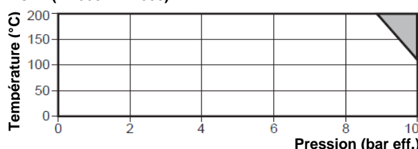
WCV1 (DN350 – DN500)
