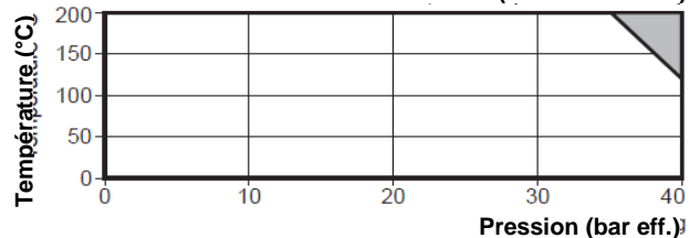
WCV3 (DN125 – DN300)
