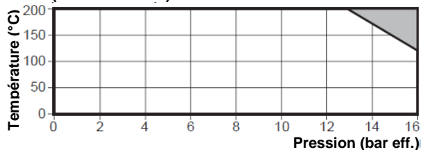
WCV1 (DN125 – DN300)
