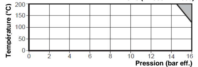
WCV3 (DN350 – DN500)
