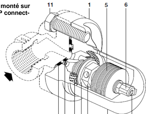
USM32 monté sur PC3_ connecteur
