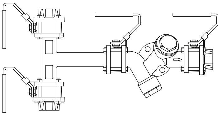
Isolement double d'équerre en amont avec robinet de purge (DBB USV)
