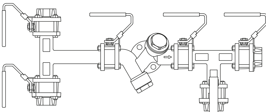
Isolement double d'équerre en amont avec robinet de purge et isolement double aval avec robinet de purge (DBB USV DSH)
