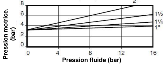
PF6_G-3BD débit au-dessus du clapet (1 à 2)
