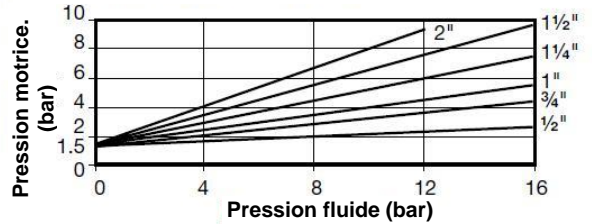
PF6_G-2NO débit au-dessous du clapet (2 à 1)
