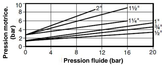
PF6_G-2NC débit au-dessus du clapet (1 à 2)
