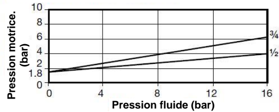
PF6_G-1NO débit au-dessous du clapet (2 à 1)
