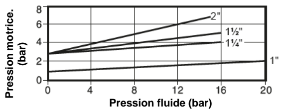
PF6_G-3NC débit au-dessus du clapet (1 à 2)
