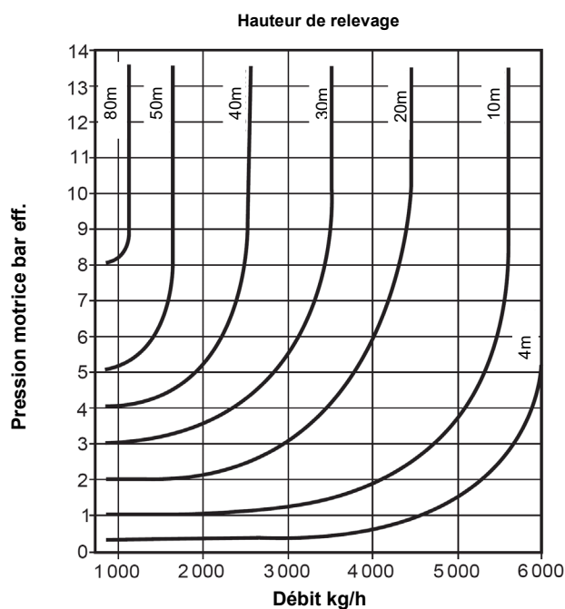
Débits de la pompe en DN80xDN50
