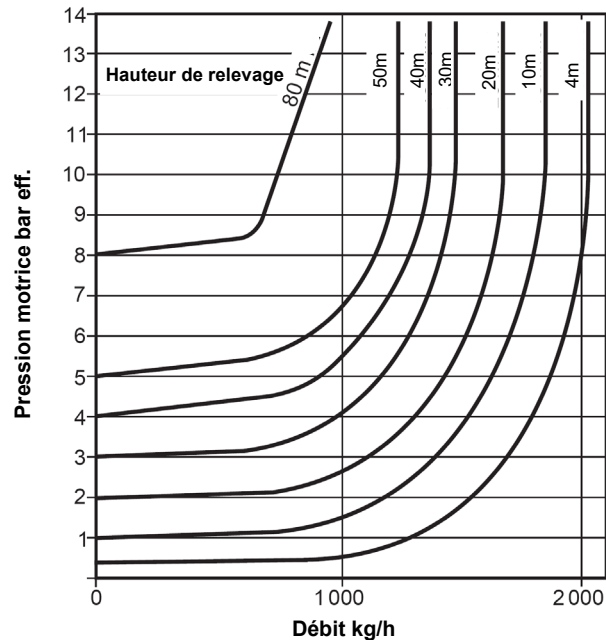
Débits de la pompe en DN40
