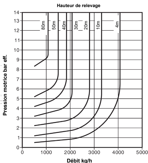
Débits de la pompe en DN50
