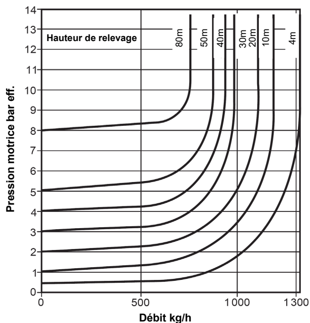
Débits de la pompe en DN25
