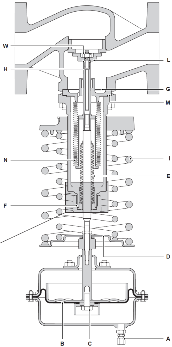
DN65 à DN100
