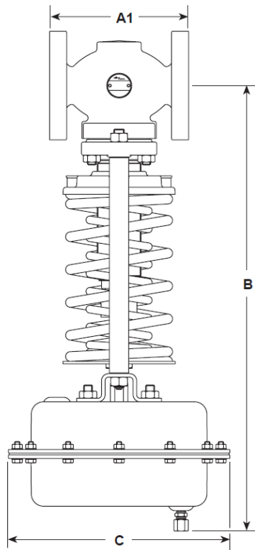
DRV-B avec actionneur type 1 ou 2
