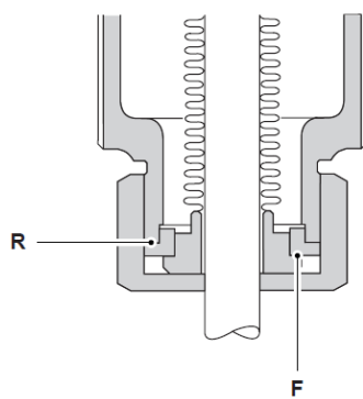
DN65 à DN100
