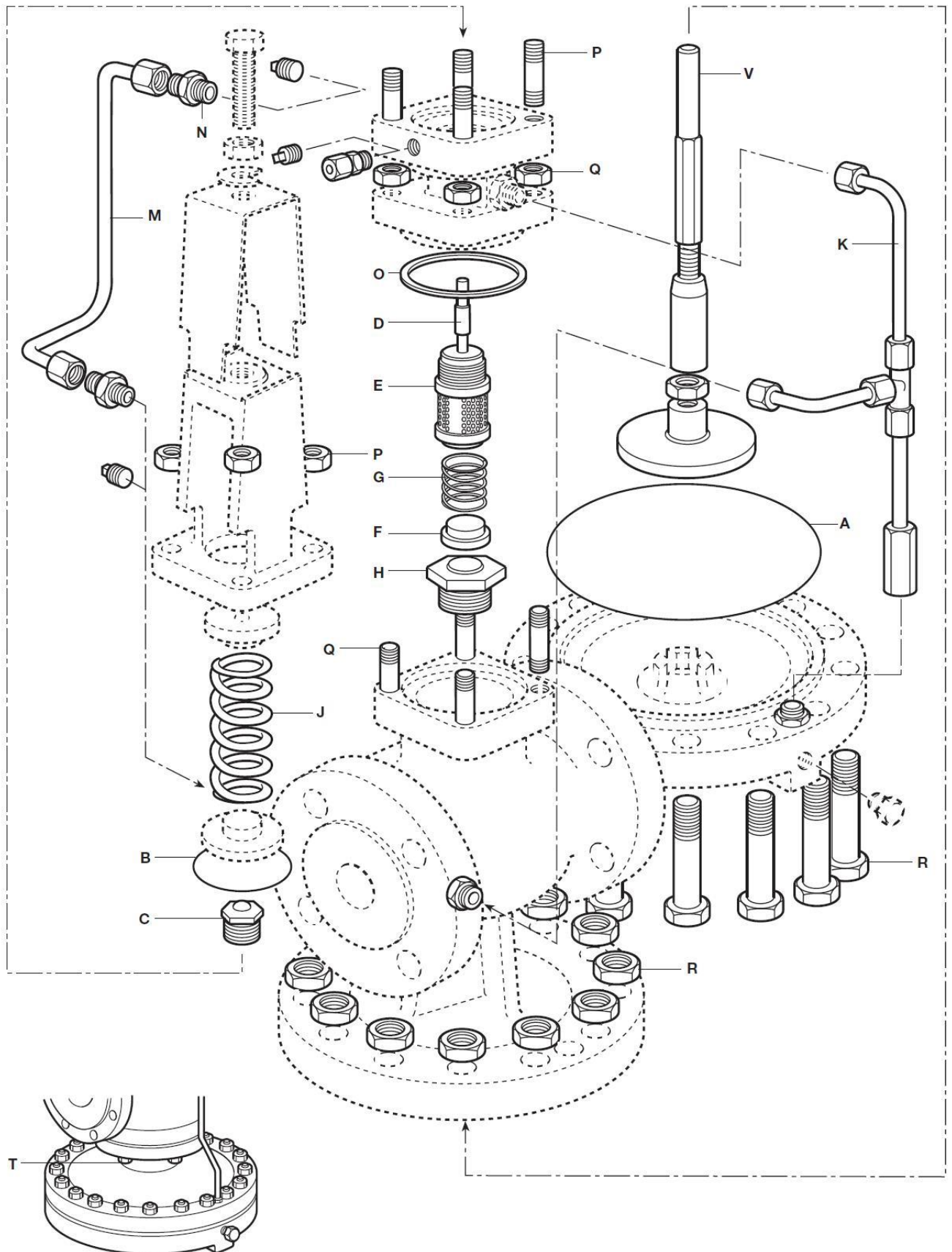
Chambre de membrane principale pour le DN80 uniquement
