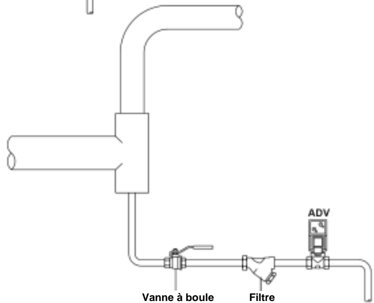
Fig.2 Purge d'un point bas
