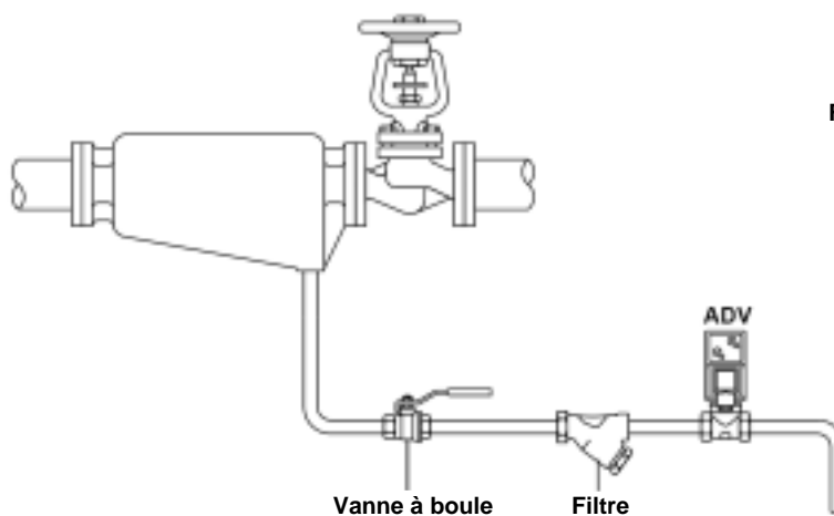
Fig.3 Purge d'un séparateur
