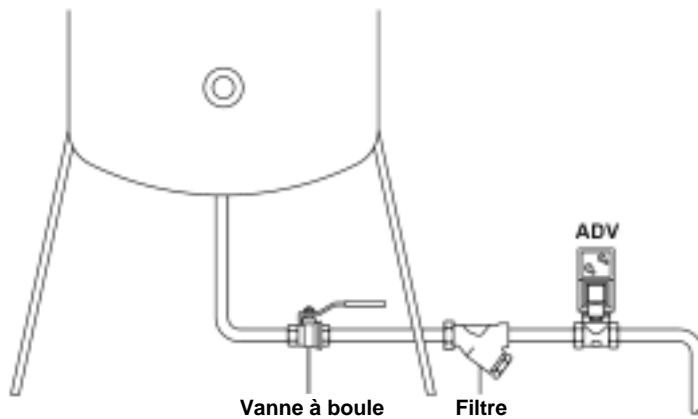
Fig.1 Purge d'un récepteur ou d'un gros filtre
