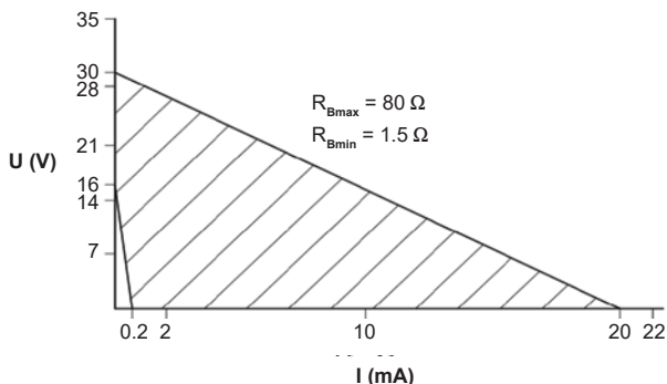
Fig. 33 - Plage de la tension et du courant d'alimentation externe
