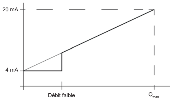
Fig. 24 - Comportement de la sortie courant
