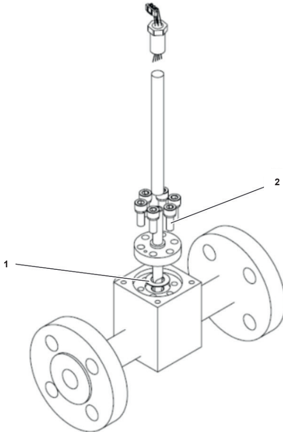
Fig. 47 - Sonde
