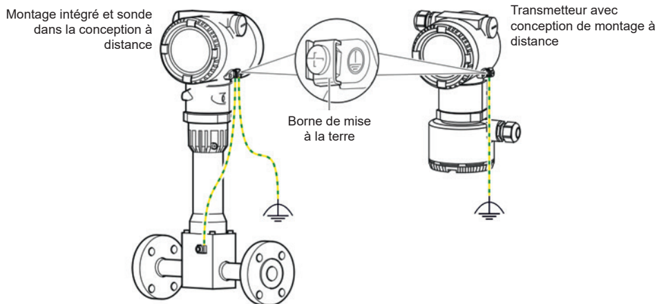
Fig. 20 - Bornes de mise à la terre
