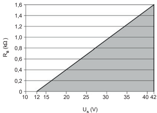
Fig. 23 - Diagramme de charge de la sortie courant ; charge en fonction de la tension d'alimentation
