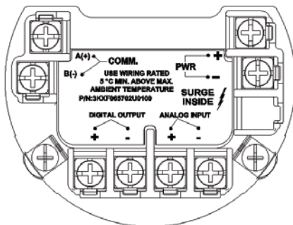
Fig. 29 - Bornes du VLM30E
