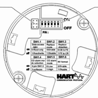
Fig. 35 - Carte de communication HART®/4 à 20 mA
