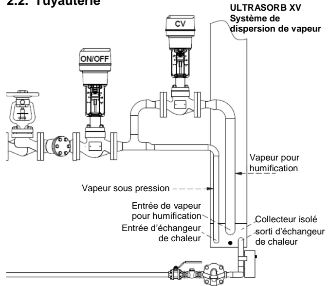
Fig. 3 Composants de tuyauterie de l'Ultra-sorb Modèle XV
