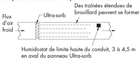
Fig. 5 Installation dans un courant d'air froid
