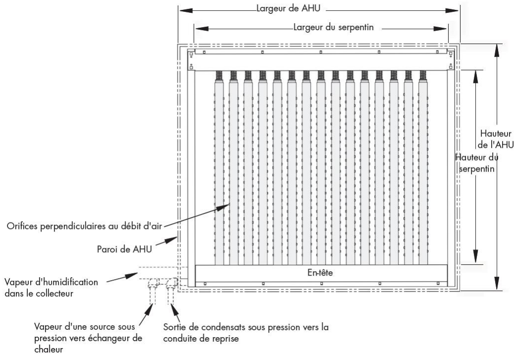
Fig. 10 Ultra-sorb Modèle XV dans une unité de traitement de l'air (flux d'air horizontal uniquement)
