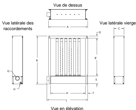
Fig. 1 - Dimensions du Ultrisorb MP
