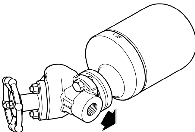
Fig. 2 - UFT14HC sur connecteur PC3_
