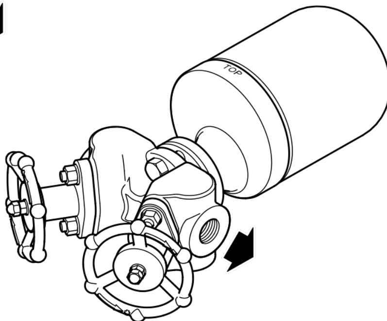
Fig. 2 - UFT14HC sur connecteur PC3_
