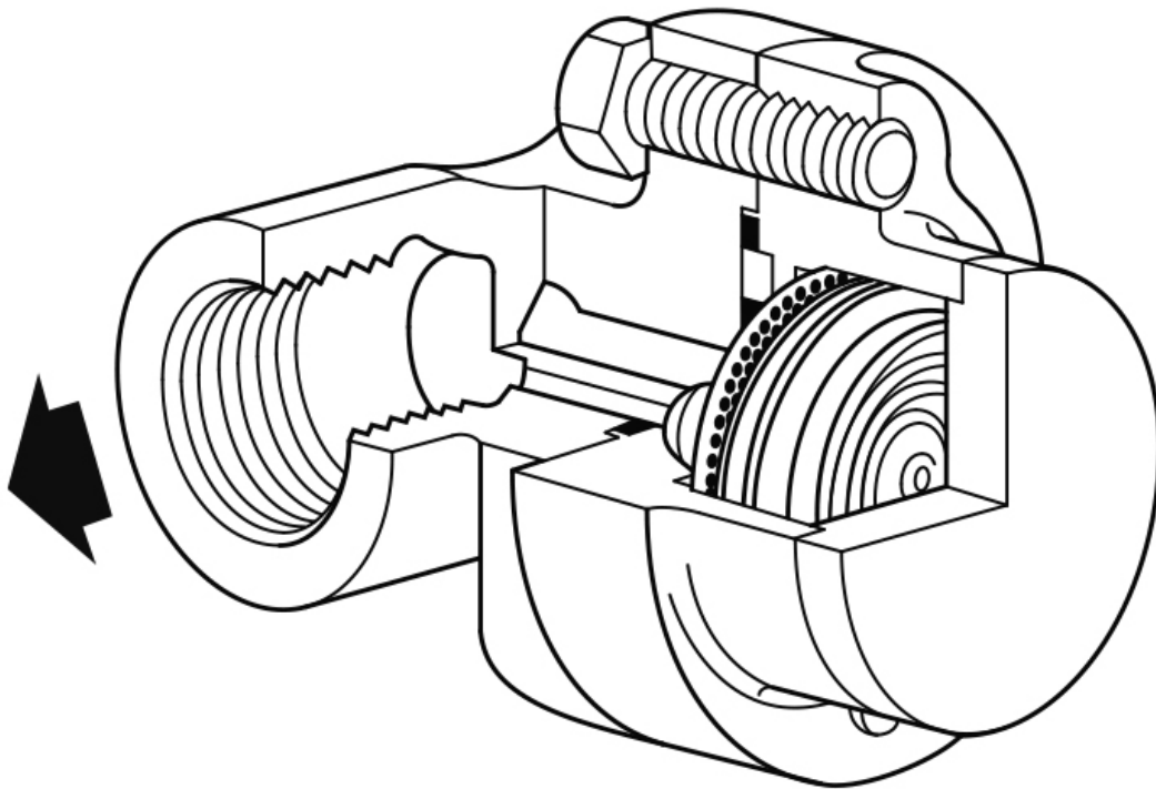
Fig. 1 - UBP32 monté sur un connecteur PC10
