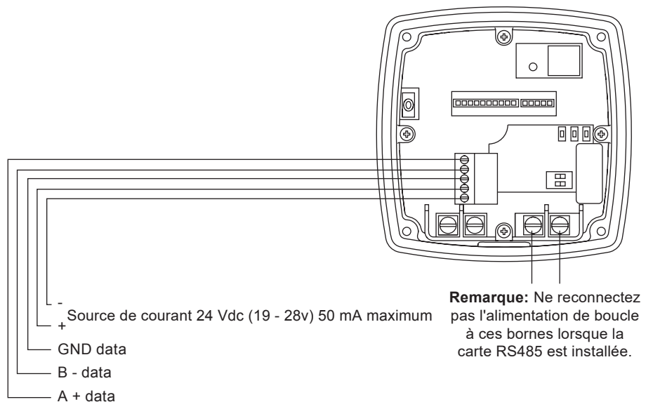
Fig. 18 TFA avec EIA 485 (RS485) Schéma de câblage des communications
