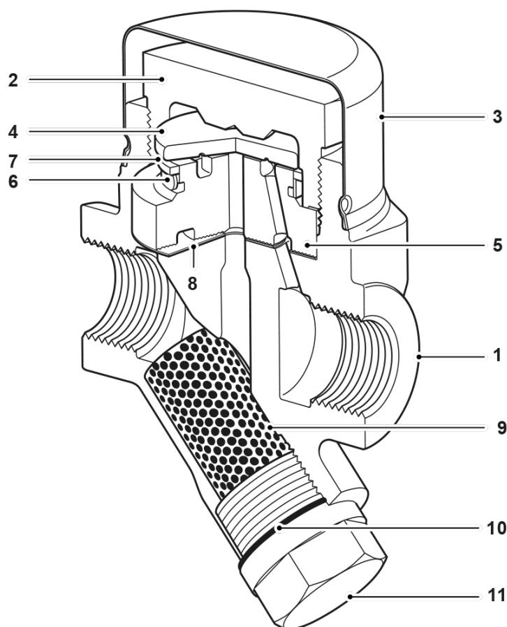
Fig. 7 - TDC46M et TDS46M Taraudés
