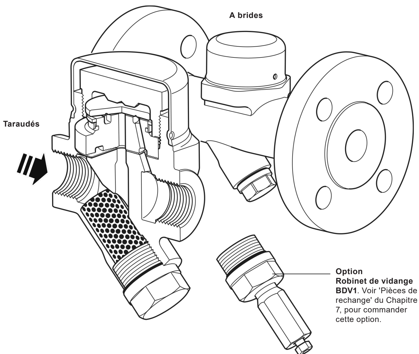
Fig. 1 - TDC46M et TDS46M - Taraudés et à brides
