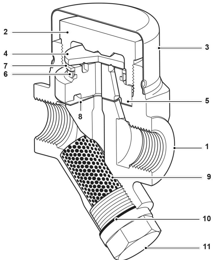
Fig. 5 - TDC46M et TDS46M Tataudés
