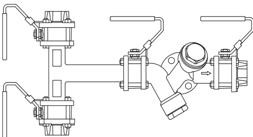
Fig. 5 - Isolement double vertical avec purge en amont
