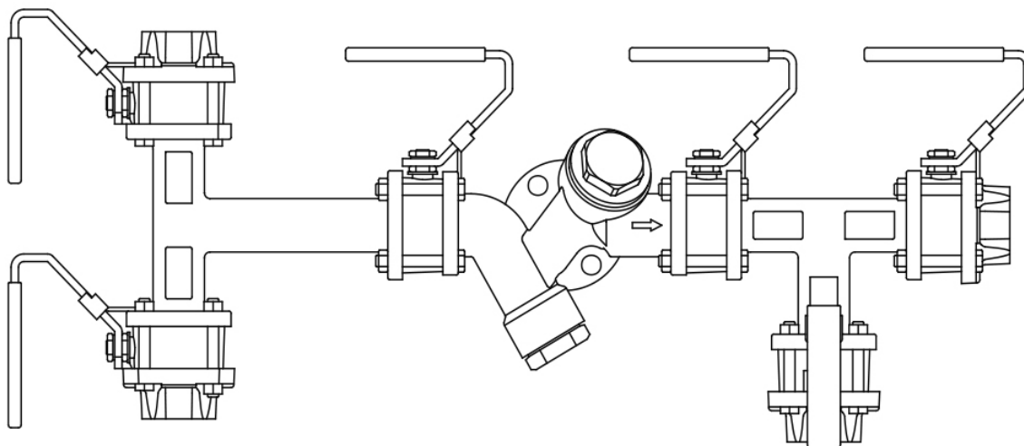
Fig. 4 - Isolement double vertical avec purge en amont et horizontal avec purge en aval
