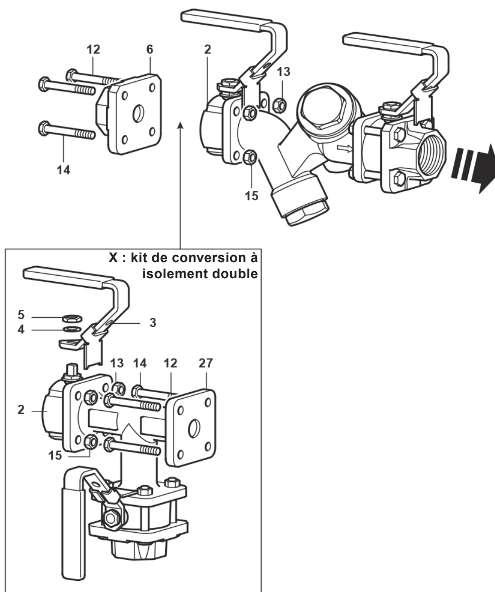
Fig. 14 - Comment monter le kit pour convertir un robinet d'isolement simple en robinet d'isolement double avec purge
