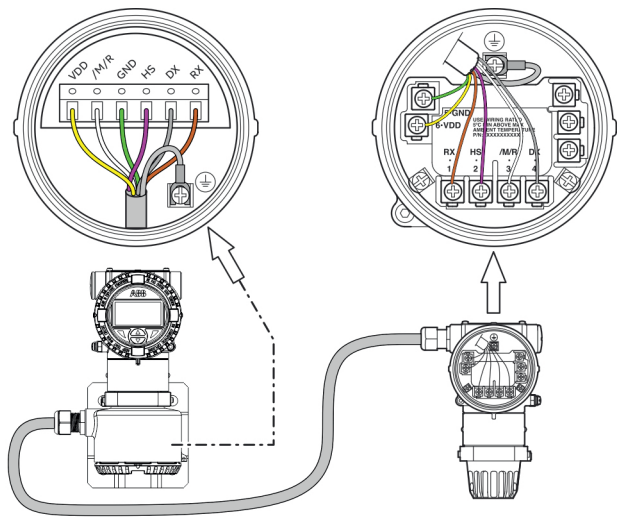
Fig. 34 - Connexion électrique
