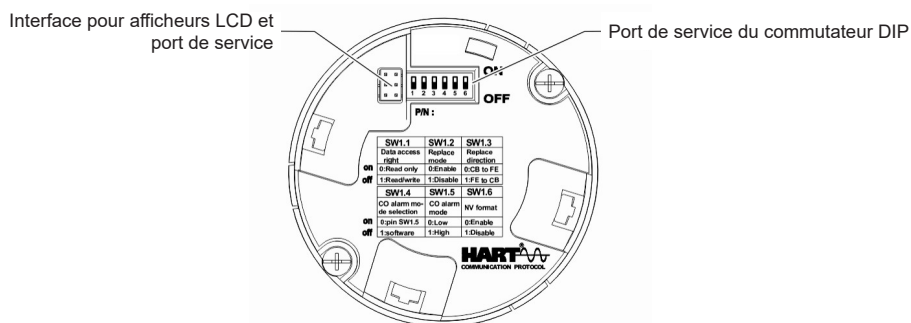
Fig. 37 - Carte de communication HART®/4 à 20 mA
