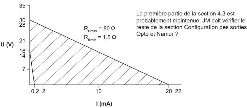
Fig. 35 - Plage de la tension et du Tension d'alimentation externe
