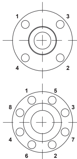
Fig. 14 - Séquence de serrage des vis de la bride
