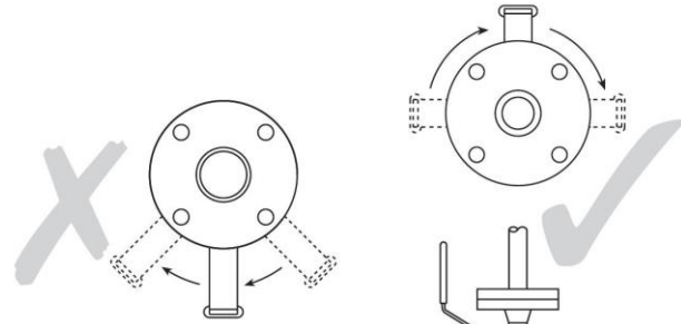
Fig. 2 Pour les liquides, le robinet ne peut pas être installé avec l'axe dirigé vers le bas.
