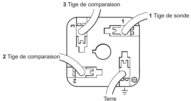
Fig. 8 Vue d'un bloc de connexion retiré du boîtier de liaison
