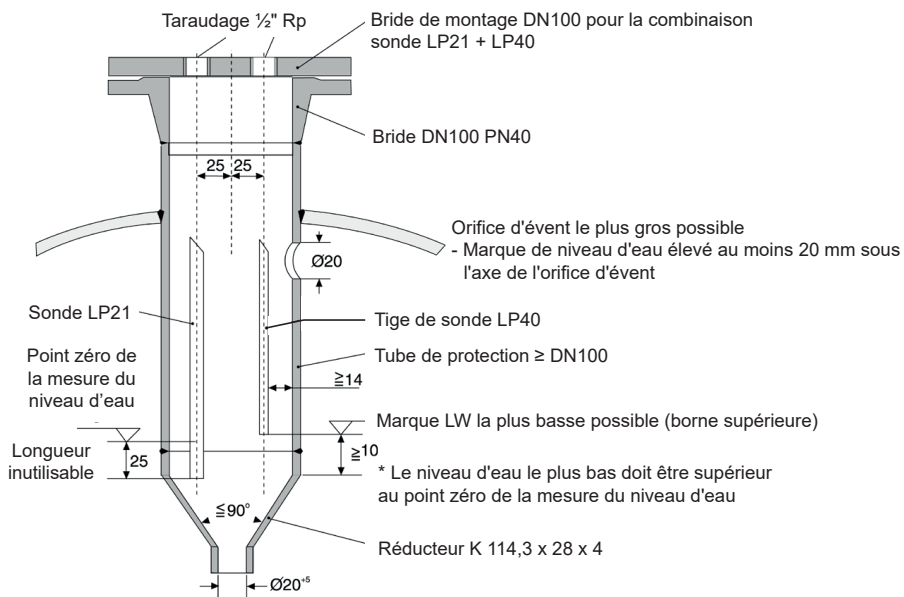
Fig. 5 Exemple d'installation 2 : Combinaison avec sonde limiteur de niveau d'eau LP40
