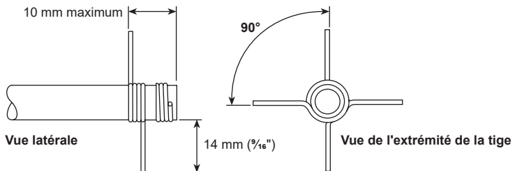
Fig. 11 Attacher (relâcher la bobine) pour le montage de la tige de sonde
