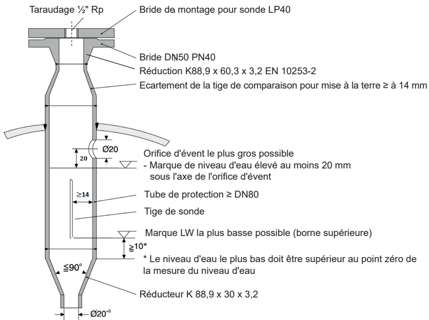
Fig. 4 Exemple d'installation 1 : À l'intérieur de la chaudière avec un tube de protection fourni par le client
