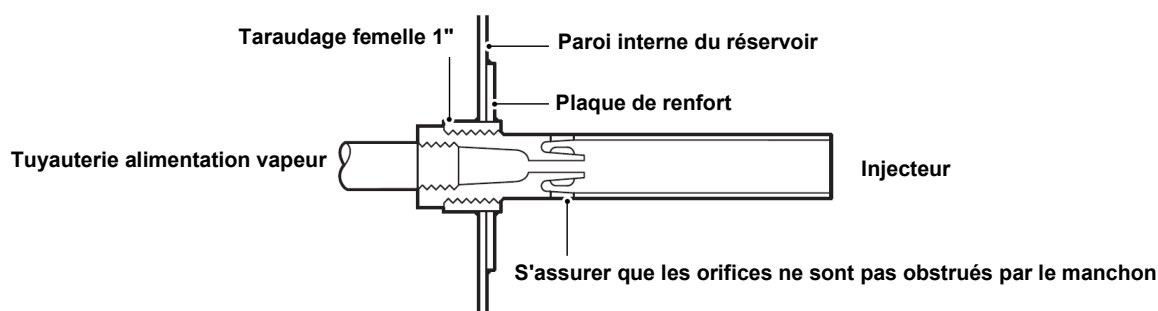
Fig. 5 IN15 – Installation typique sur une paroi du réservoir
