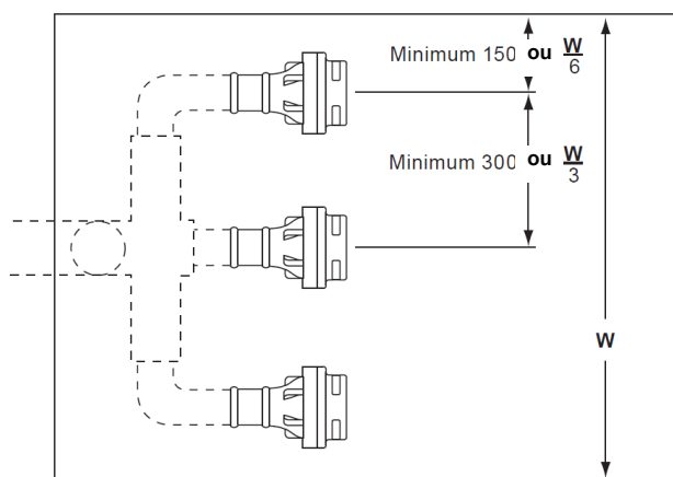
Fig. 8 Trois injecteurs
