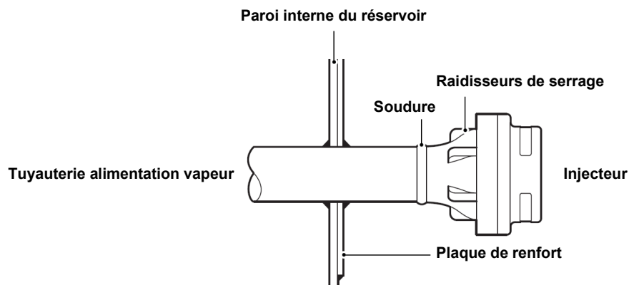
Fig. 4 IN25M/IN40M – A souder BW - Installation typique sur une paroi du réservoir (sur tube soudé)
