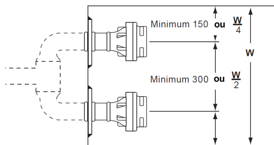
Fig. 7 Deux injecteurs
