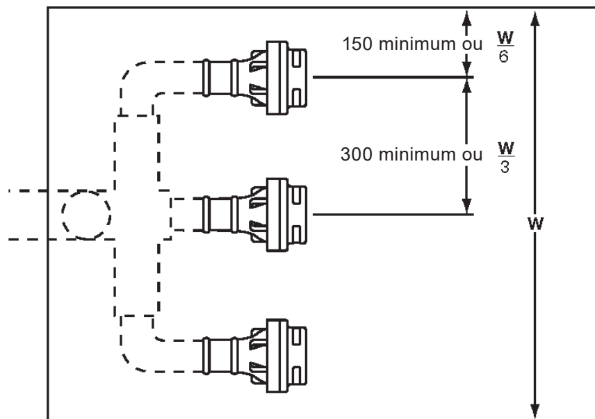
Fig. 8 Position de trois buses
