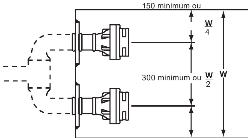
Fig. 7 Position de deux buses
