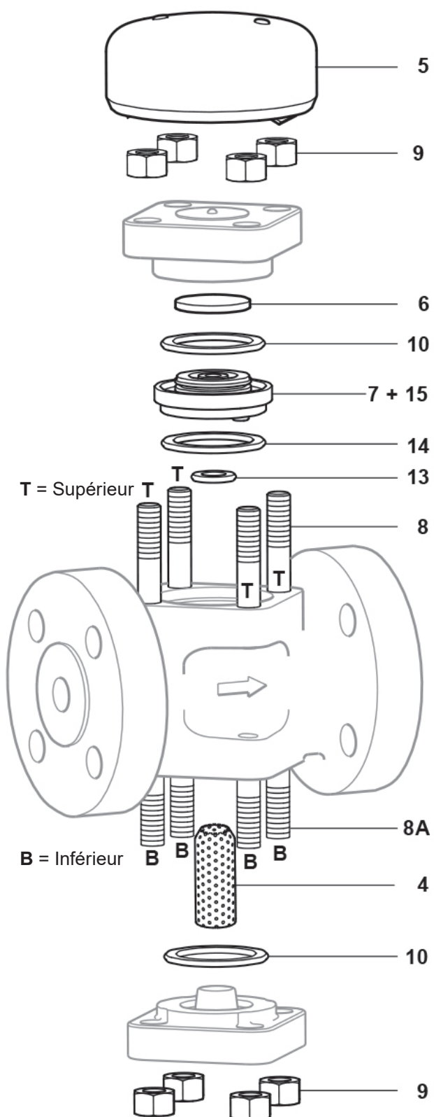
Fig. 13 - Versions à brides
