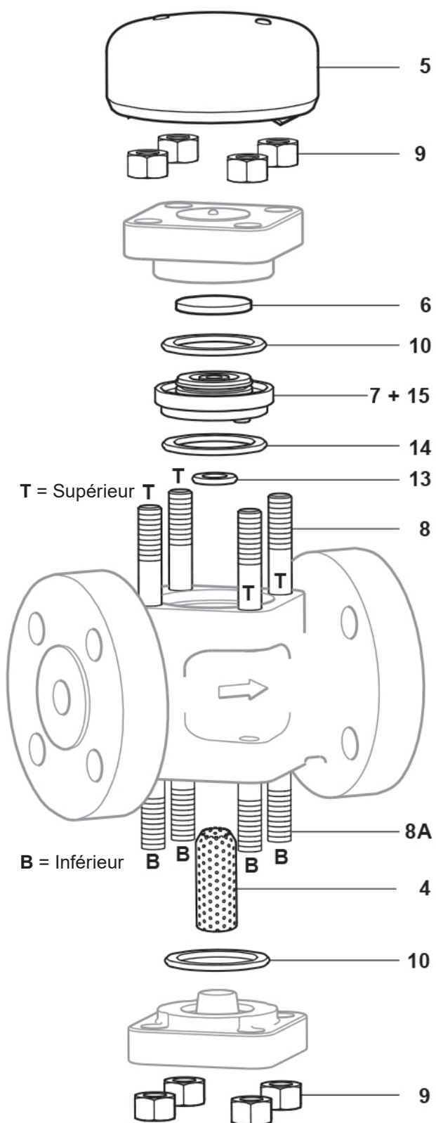
Fig. 10 - Versions à brides
