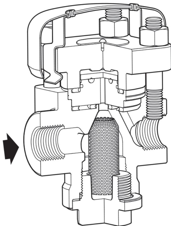
Fig. 1 - Taraudé/à souder socket-weld
