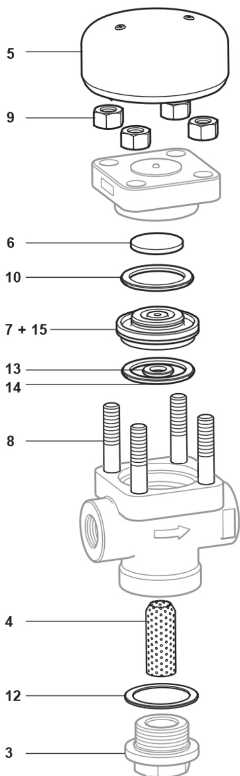
Fig. 12 - Versions taraudées et socket-weld
