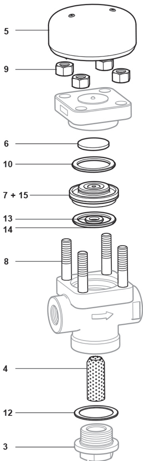
Fig. 9 - Versions taraudées et socket-weld
