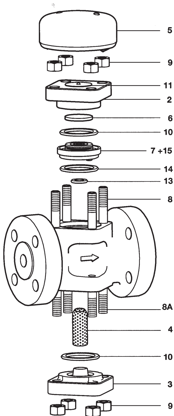
Fig. 8 - Versions à brides
