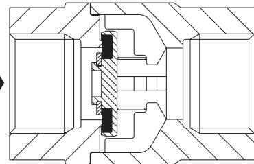
Fig. 2 - Option portée souple (uniquement pour la version taraudée)
