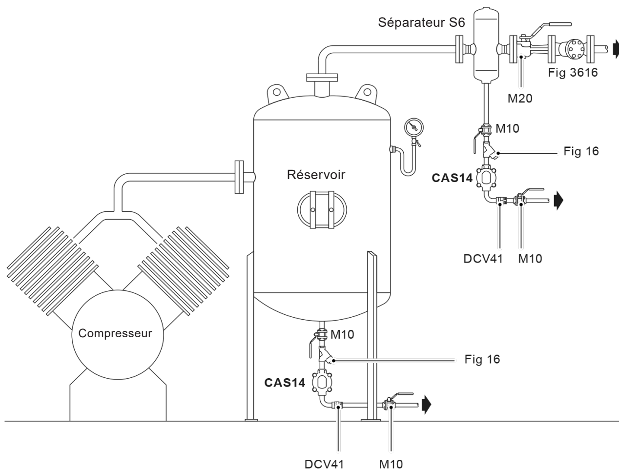
Fig. 3 - Installation typique
