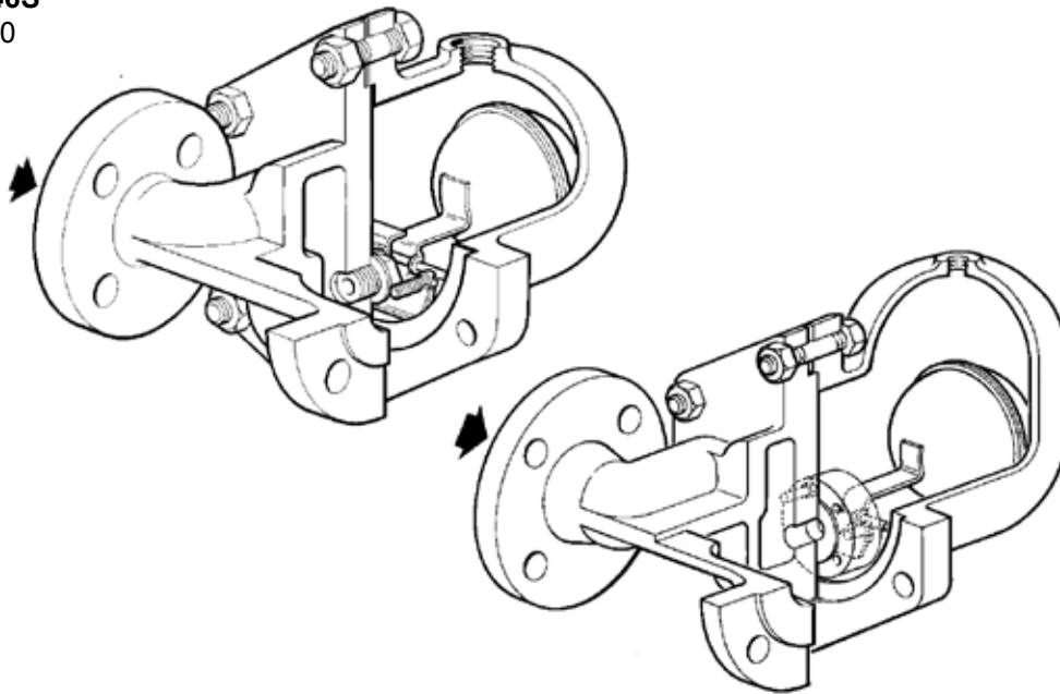
Fig. 4 CA46S DN40 et DN50 à brides EN
