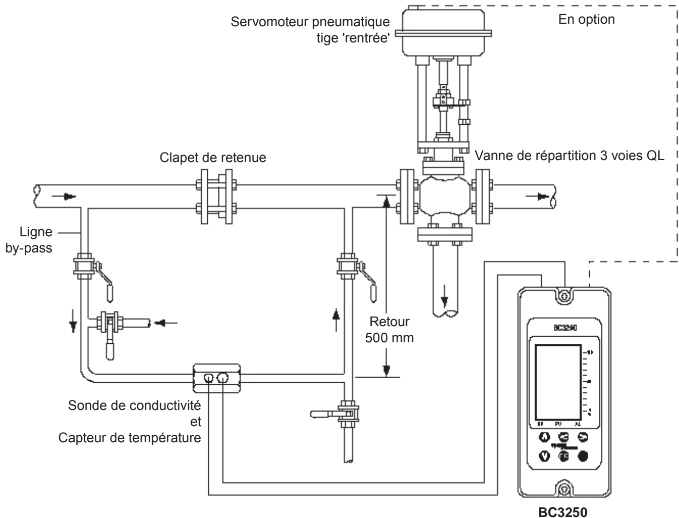
Fig. 13 Système CCD
