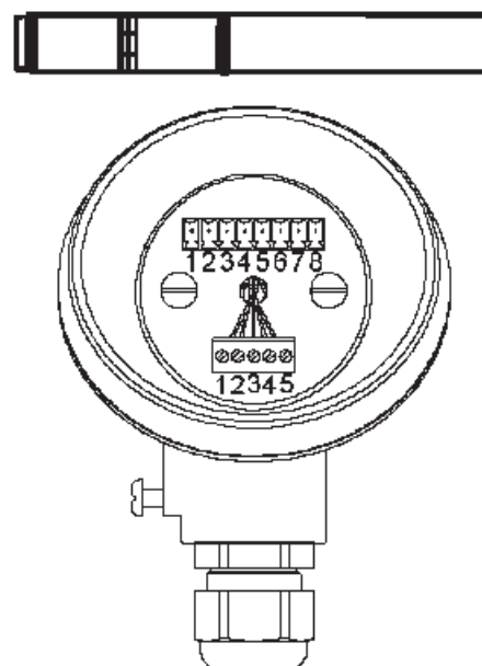
Fig. 26 Ancien modèle de CP32 (sans circuit pulsé) Sélectionner : 'PULSED'
