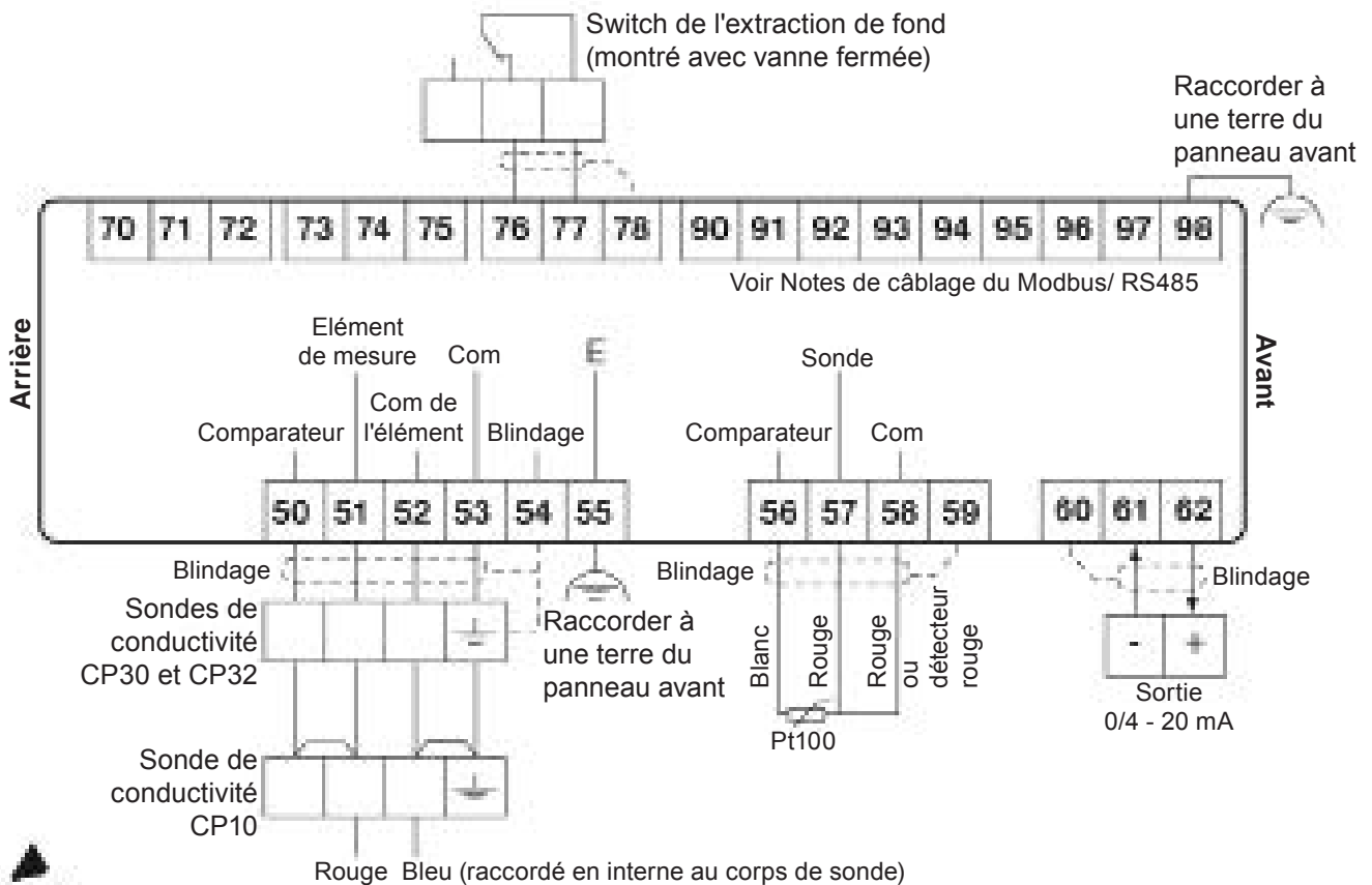
Fig. 20 Circuit de branchement (vue d'en haut)
