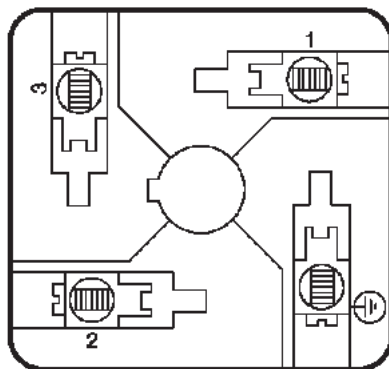
Fig. 19 Vue du bloc de connexion du CP30
