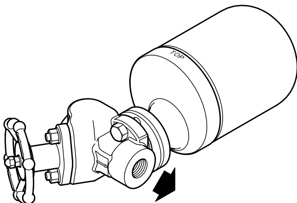
Fig. 2 UFT14HC montado en el conector PC3_
