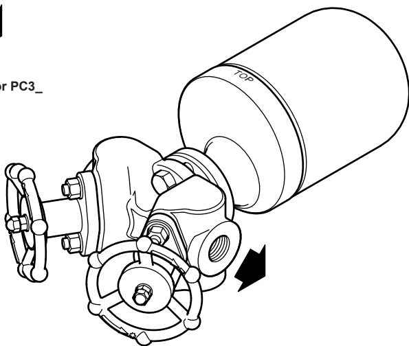
Fig. 3 UFT14HC montado en el conector PC4_
