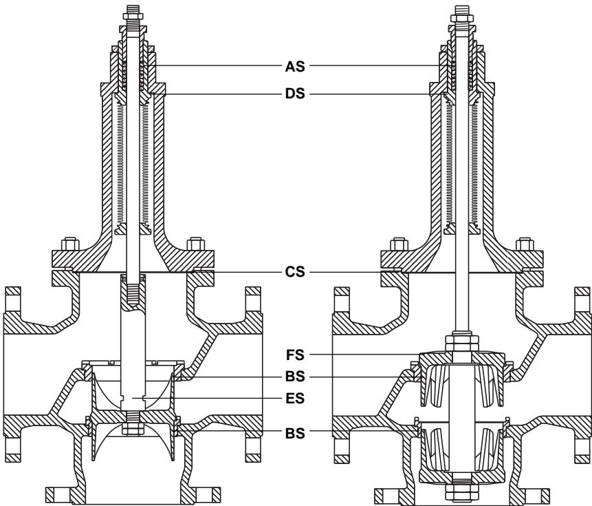
Válvula mezcladora
