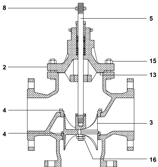
Fig. 7 Válvula mezcladora
