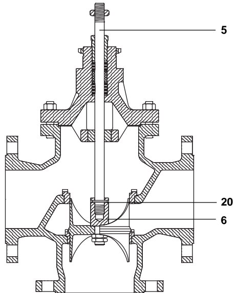
Fig. 5 Válvula mezcladora
