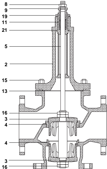
Fig. 11 Válvula desviadora
