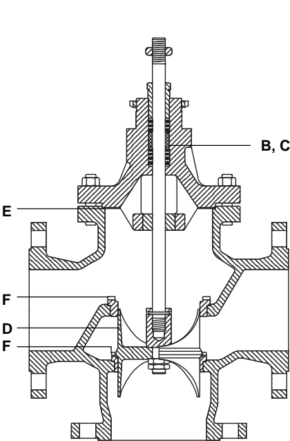
Válvula mezcladora
