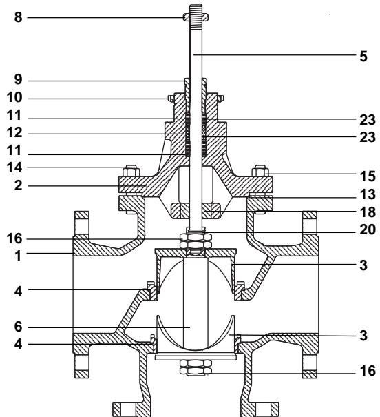
Fig. 2 Válvula desviadora
