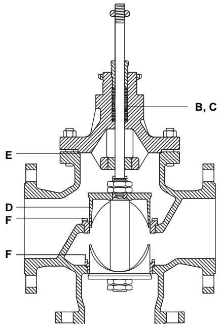
Válvula desviadora
