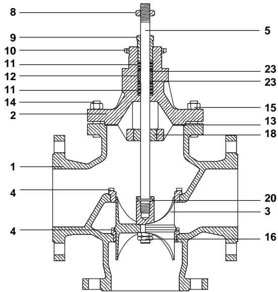
Fig. 1 Válvula mezcladora
