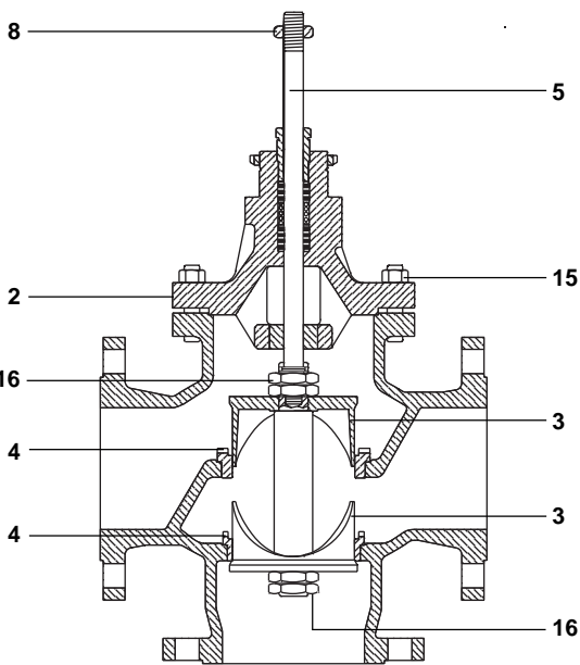
Fig. 8 Válvula desviadora
