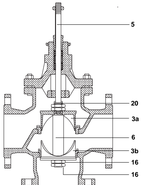
Fig. 6 Válvula desviadora
