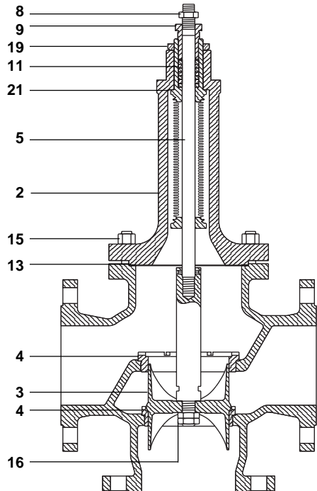
Fig. 10 Válvula mezcladora
