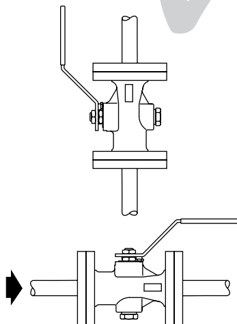
Fig. 3 Instalación correcta para trabajar con gases
