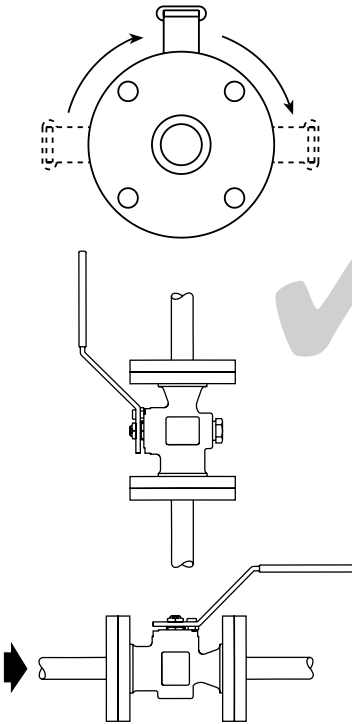
Fig. 3 Instalación correcta para servicio con gas
