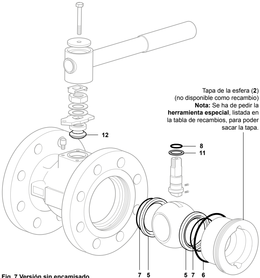
Fig. 7 Versión sin encamisado.
