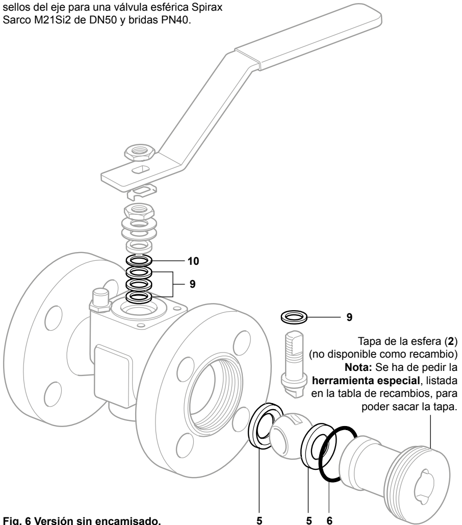
Fig. 6 Versión sin encamisado.
