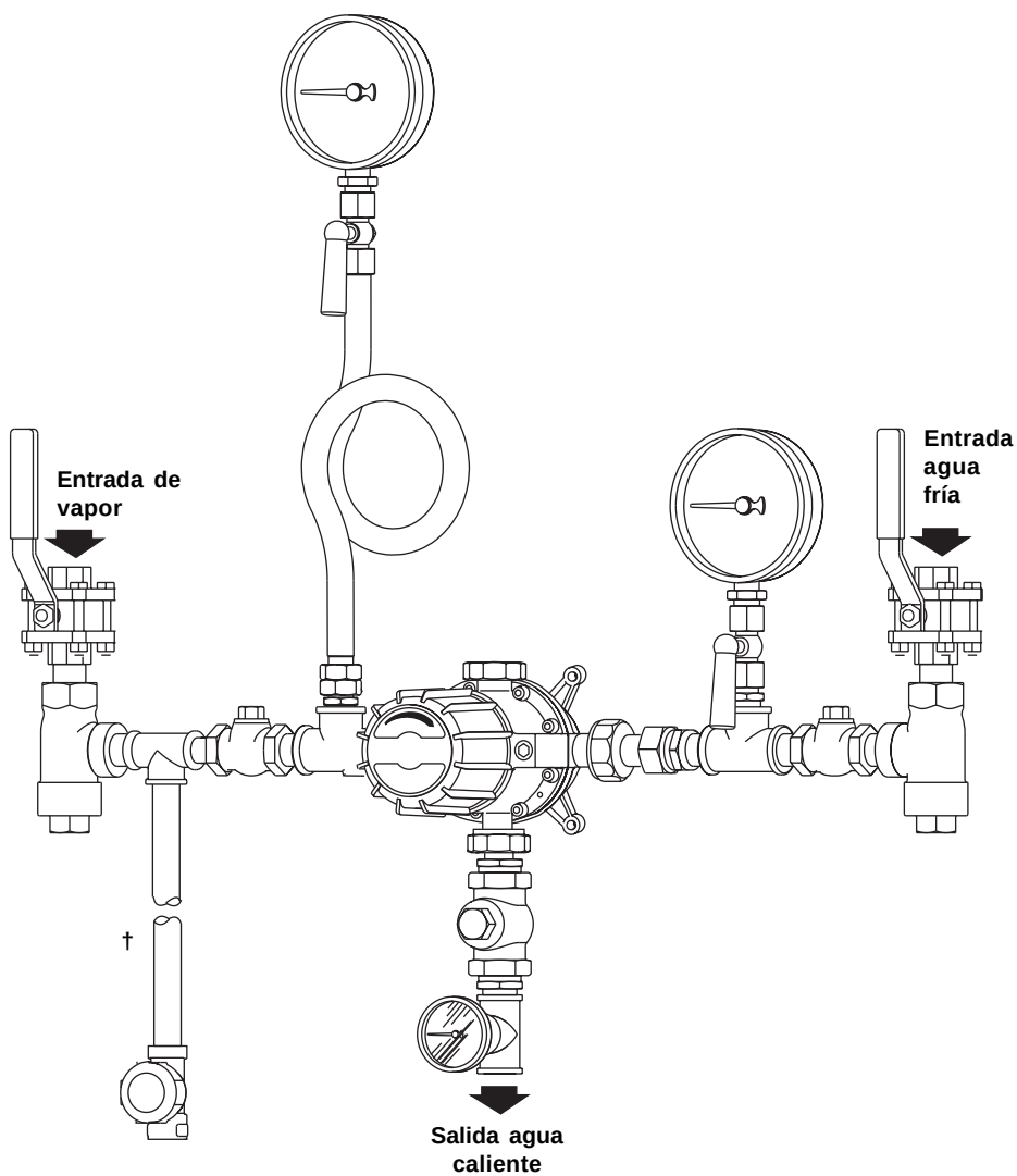
Fig. 1 Estación de ½" y ¾"
