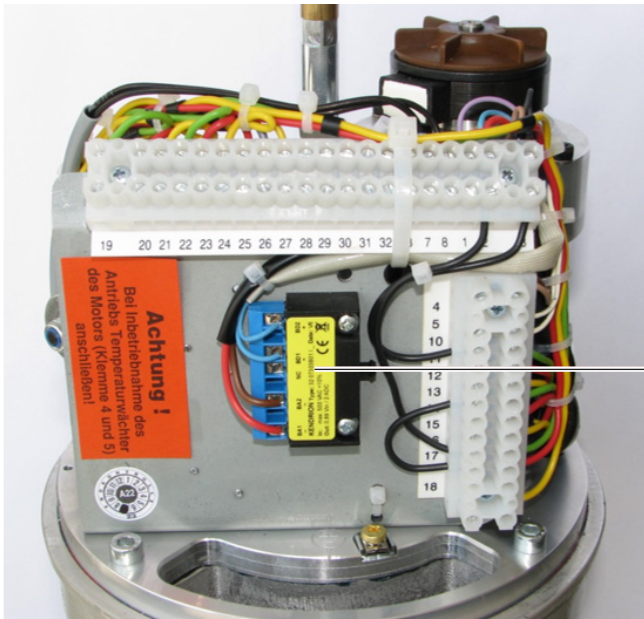
Fig. 21 Instalación del calefactor anti-condensación (8-20 kN)
