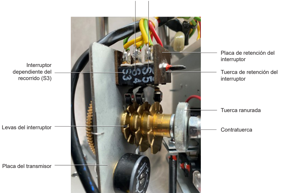
Fig. 10 Disposición del interruptor de recorrido auxiliar (WE) (8 kN+)
