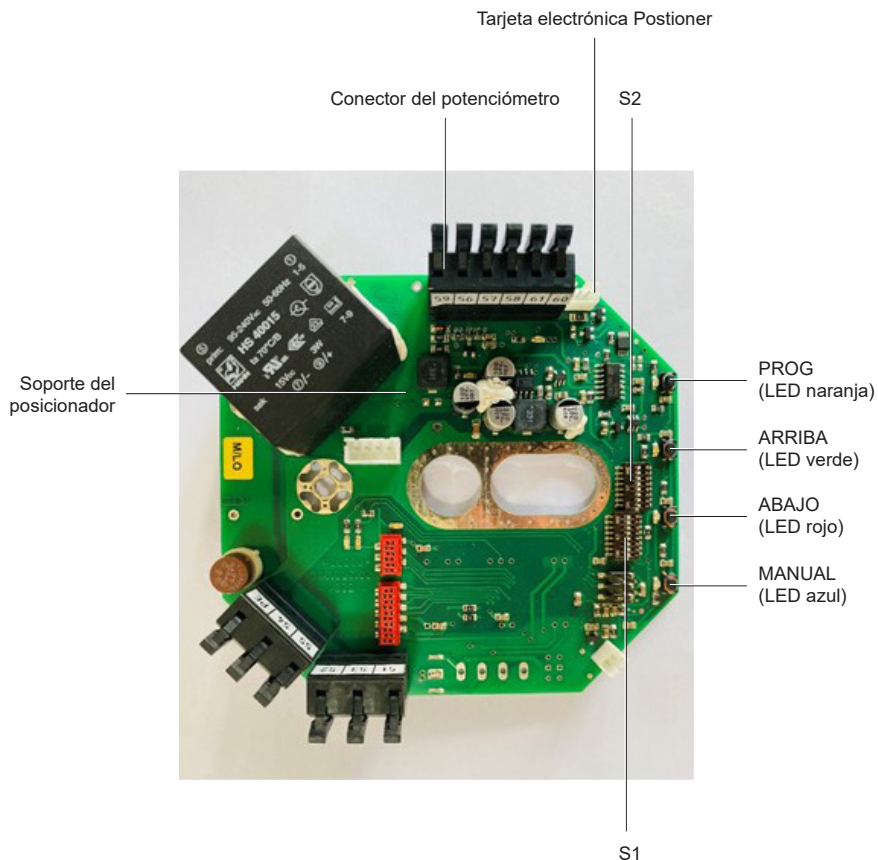
Fig. 28 Tarjeta Electrónica del Posicionador Vac
