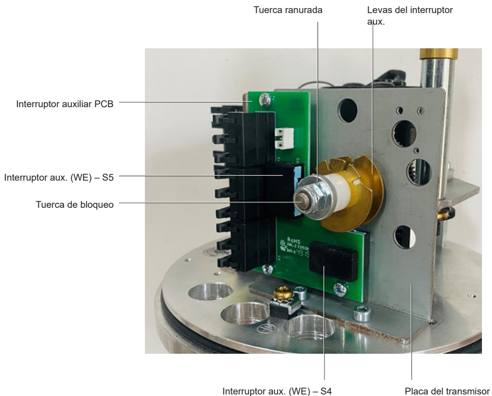
Fig. 9 Disposición del interruptor de recorrido auxiliar (WE) (1-6 kN)
