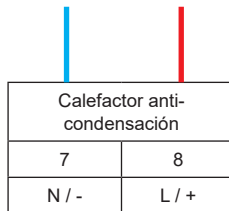
Fig. 23 Esquema de terminales del calefactor anti-condensación
