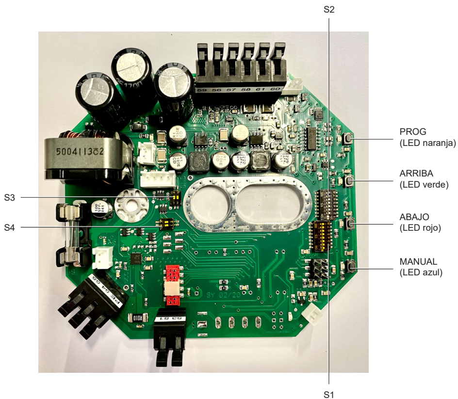
Fig. 29 Tarjeta electrónica del posicionador Vcc (incluidas las versiones del módulo de desconexión)
