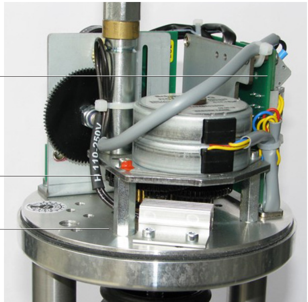
Fig. 16 Instalación del calefactor anti-condensación (1 kN)
