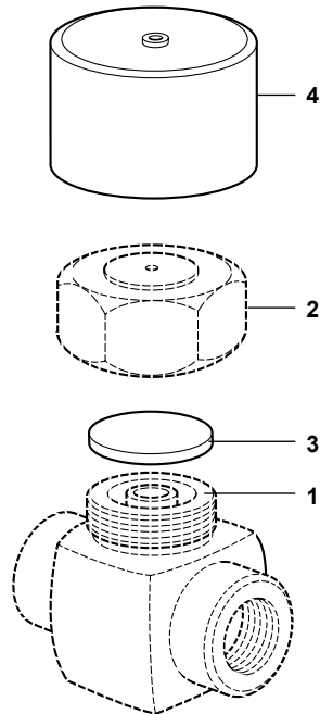
Fig. 4 TD52M shown
