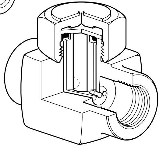
Fig. 2 TD52M
