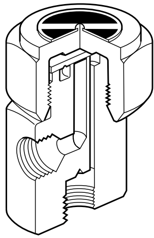
Fig. 3 TD259
